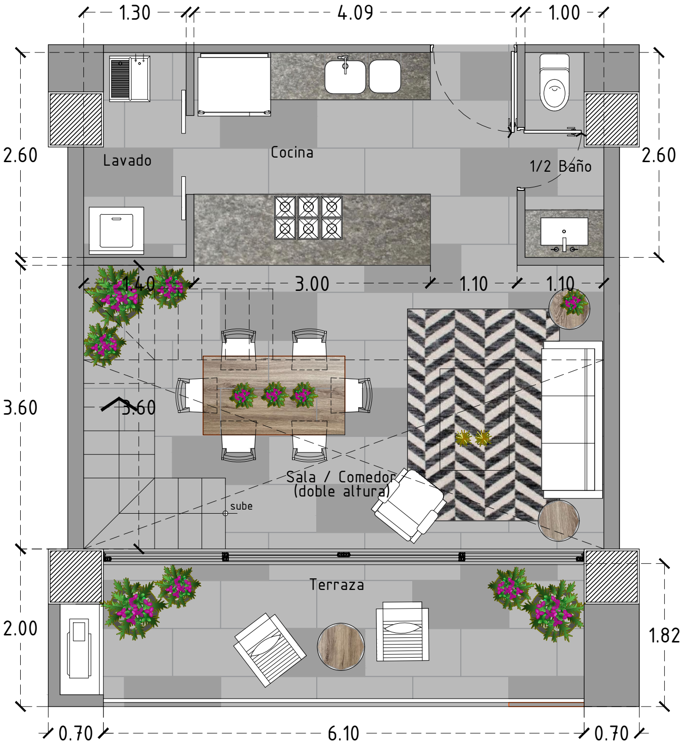
PLANTA BAJA
